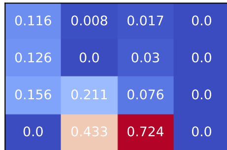
Value function v^*(s)
